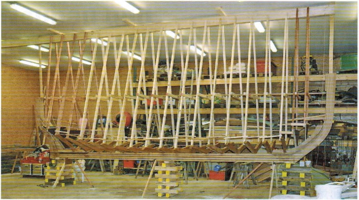
In Bad Bederkesa entsteht gegenwärtig auch ein Neubau. Die Kiellegung des Acht-Meter-Bootes erfolgte am 8. Dezember. Mit der Fertigstellung wird zur Saison 2019 gerechnet.
